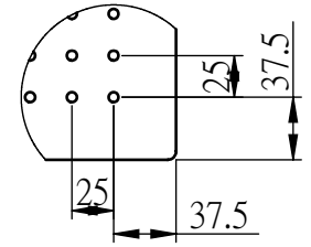
細部放大圖 B 比例 1 : 5
