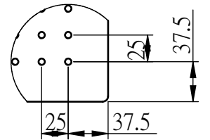
細部放大圖 B 比例 1 : 5
