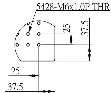
細部放大圖 A 比例 1 : 5
