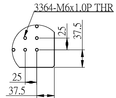
細部放大圖 A 比例 1 : 5
