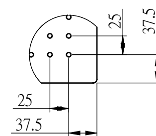
細部放大圖 A 比例 1:5
