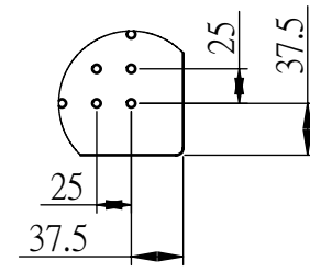
細部放大圖 A 比例 1:6
