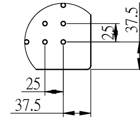
細部放大圖 A 比例 1:5
