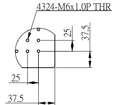
細部放大圖 A 比例 1 : 5
