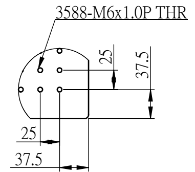
細部放大圖 A 比例 1 : 5
