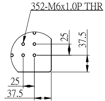
細部放大圖 A 比例 1:5
