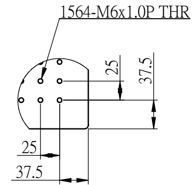
細部放大圖 A 比例 1 : 5
